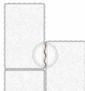
Nűtfédes térkövek kapcsolódása
