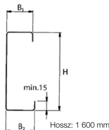
CI GERENDA
